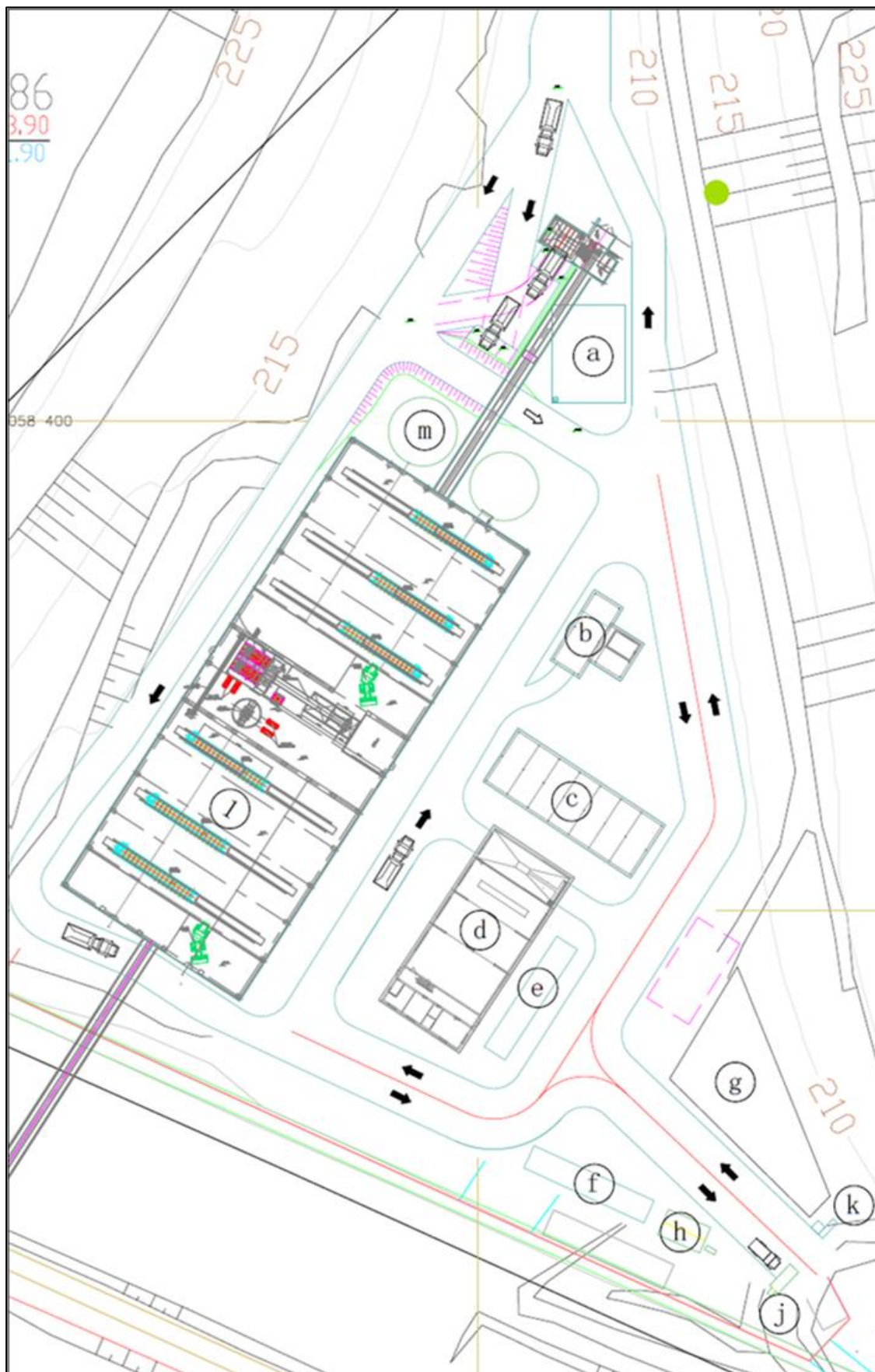
Obrázek č. 36: Schéma umístění stavebních objektů v zázemí lomu
